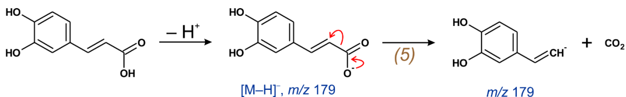
Rysunek 8. Ścieżki fragmentacji kwasu kawowego zachodzące dla jonu [\text{M} - \text{H}]^- ( m/z 179)
